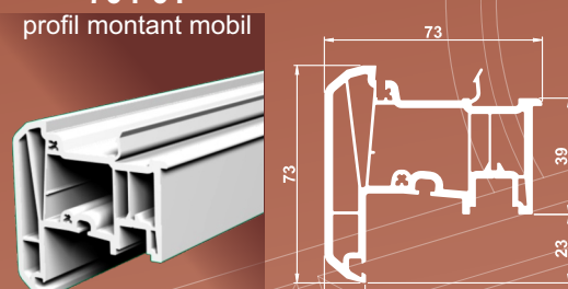
704-01 profil montant mobil
