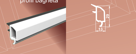
605-02 profil baghetă
