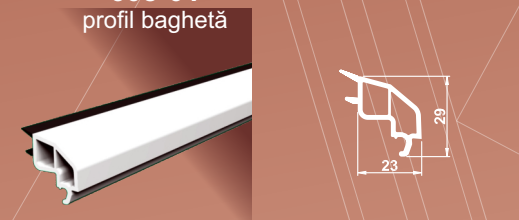
605-01 profil bagheta
