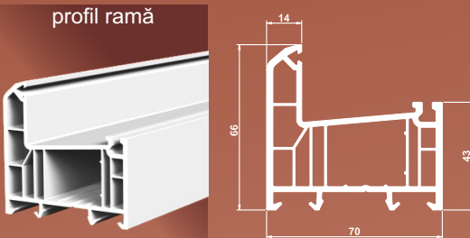
701-01 profil ramă
