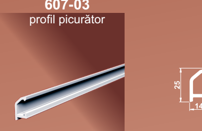
607-03 profil picurător
