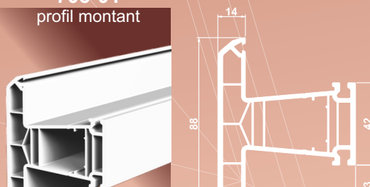
703-01 profil montant
