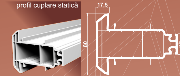
606-06 profil cuplare statică
