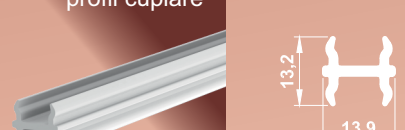
306-01 profil cuplare
