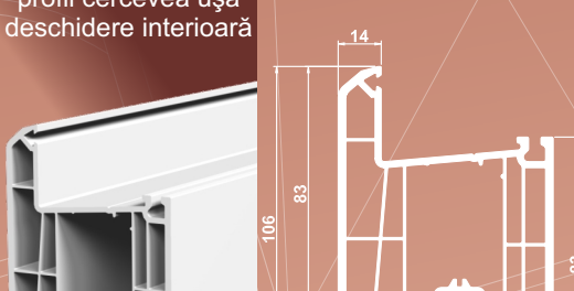
702-02 profil cercevea ușă deschidere interioară
