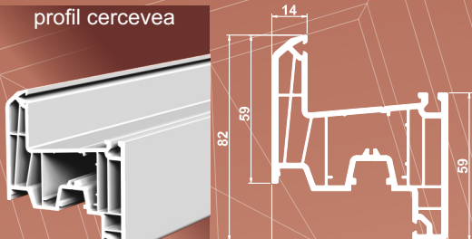
702-01 profil cercevea
