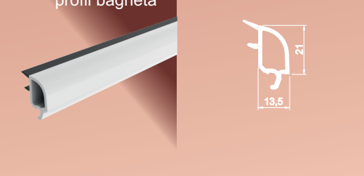
605-03 profil baghetă
