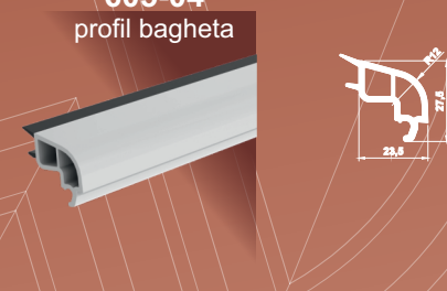
605-04 profil bagheta
